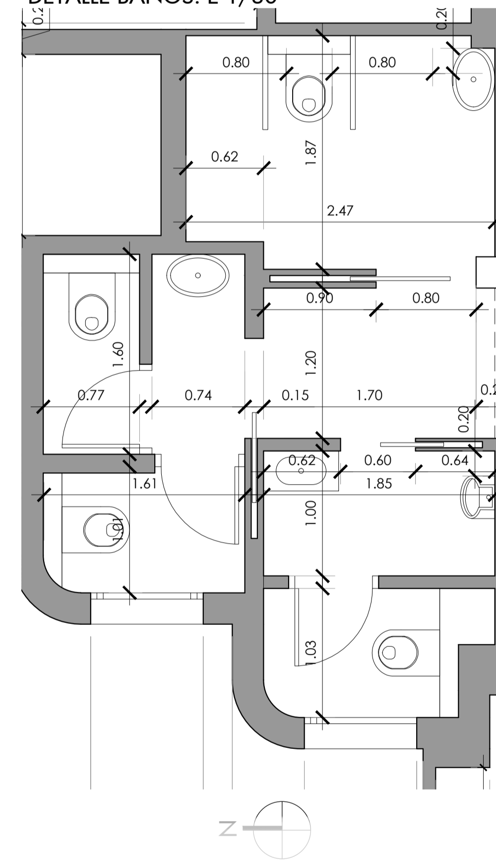
DETALLE BAÑOS. E 1/30
