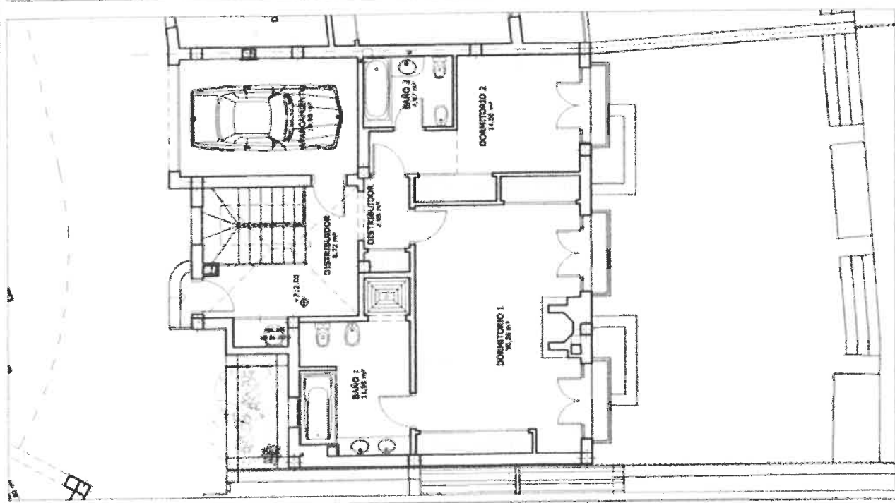
PLANTA A COTA +212.00 m
