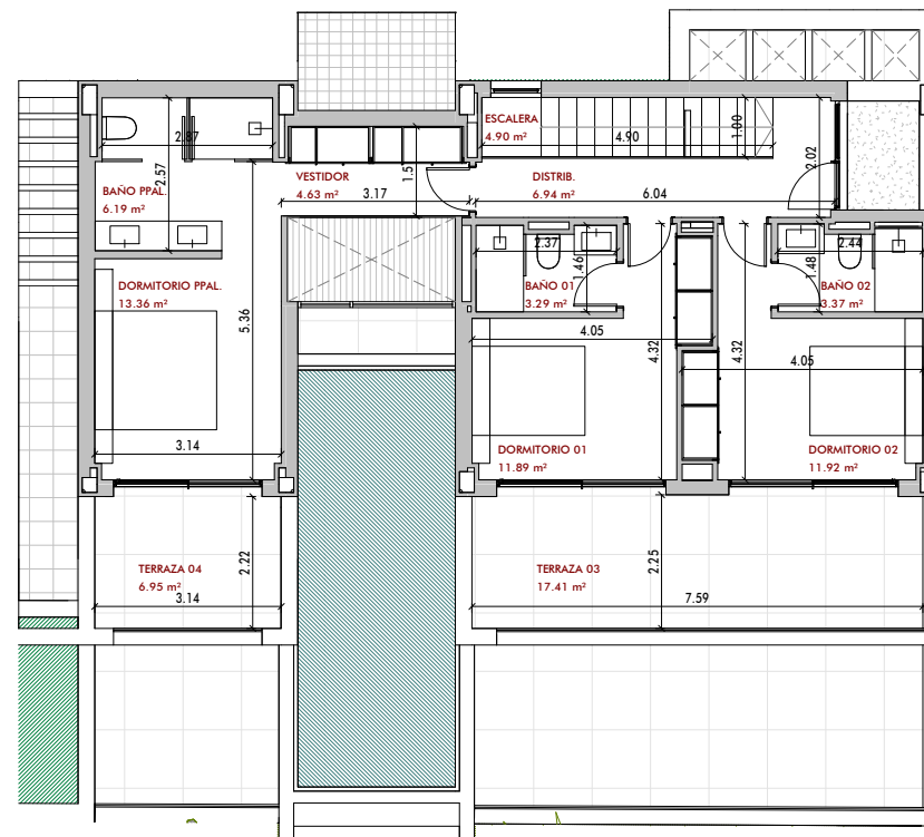
PLANTA PRIMERA
