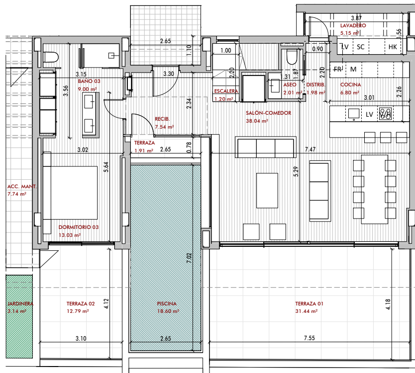
PLANTA ACCESO
