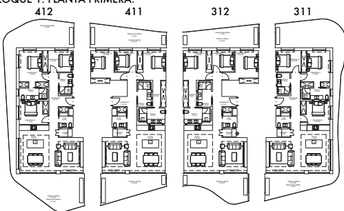
BLOQUE 1. PLANTA PRIMERA. 412
