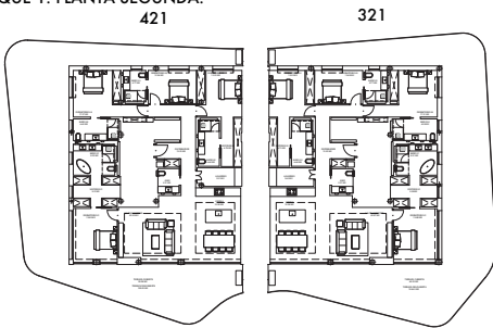
BLOQUE 1. PLANTA SEGUNDA. 421
