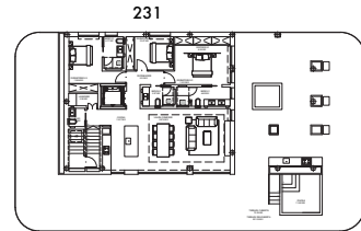
BLOQUE 2. PLANTA ÁTICO.
