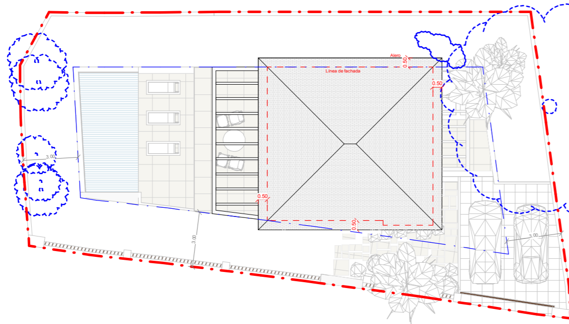
4 PLANTA DE CUBIERTAS B05 1:100
