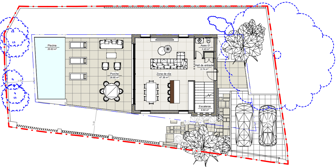
2 PLANTA BAJA B05 1:100
