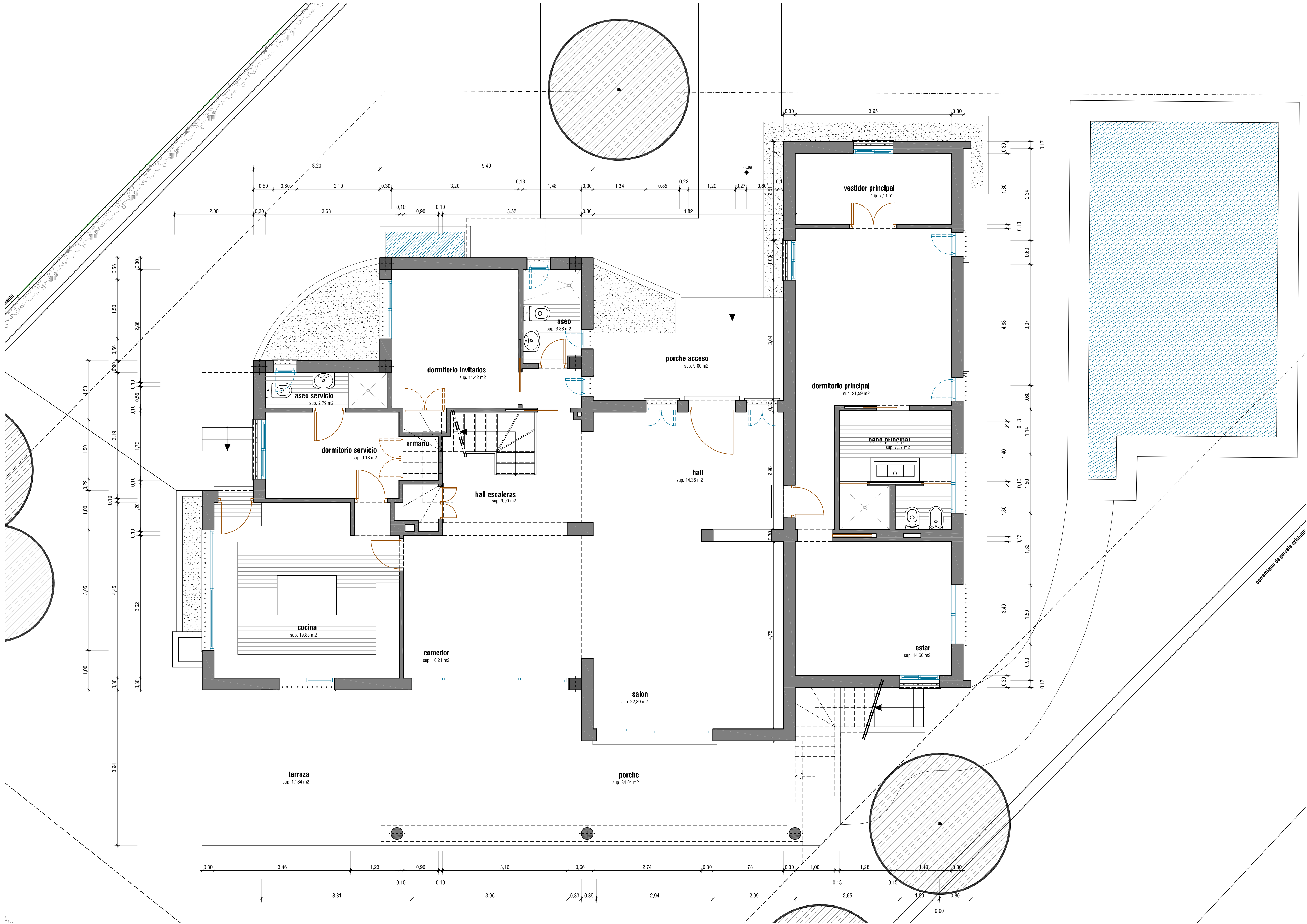
planta baja - estado reformado E1/50
