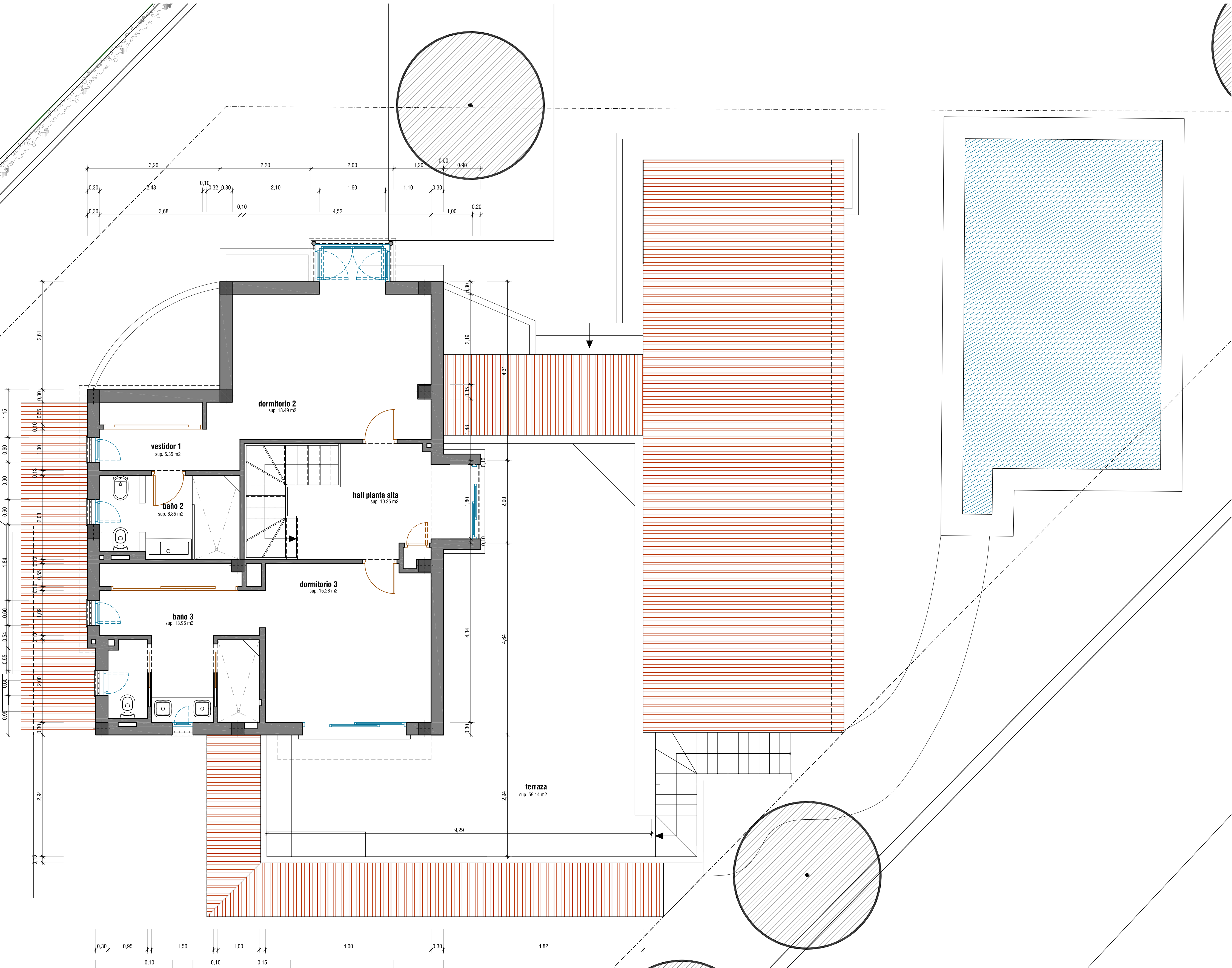
planta alta - estado reformado E1/50
