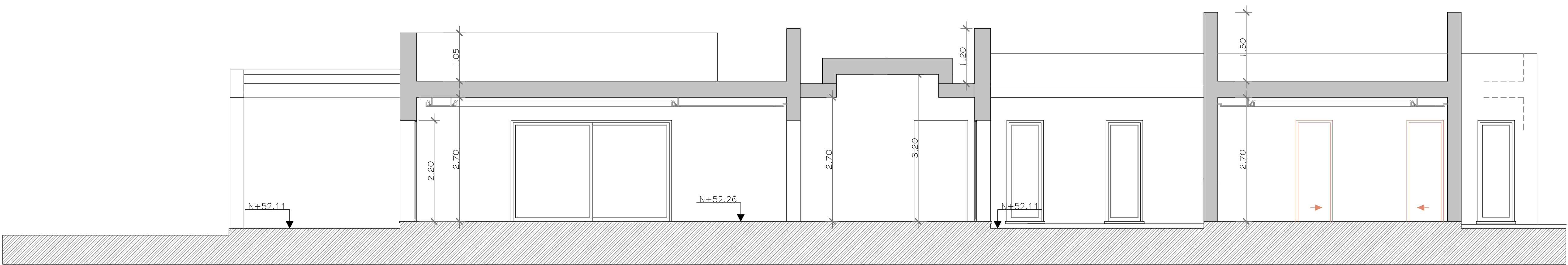
SECCION C-D
