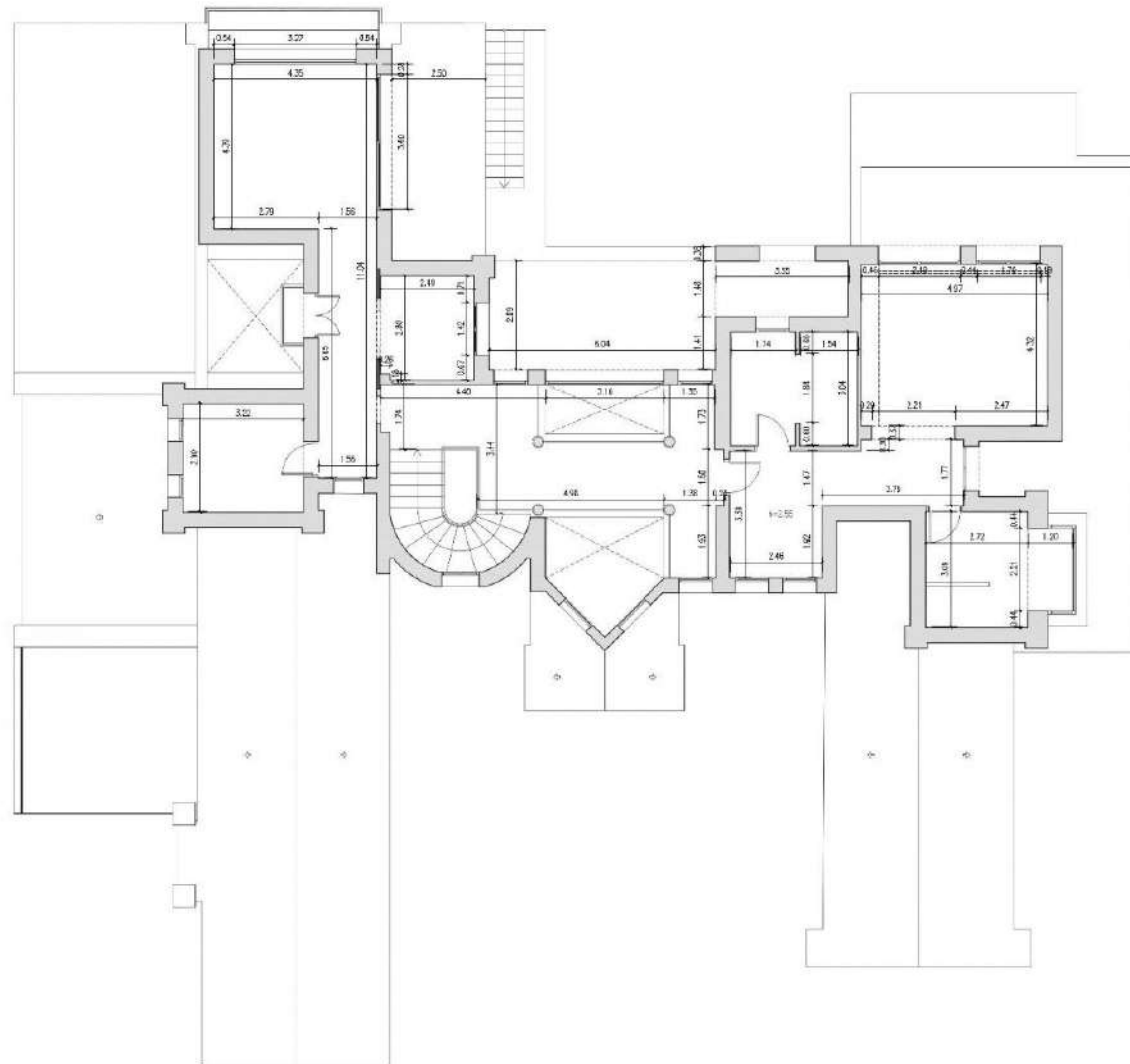
VILLA LOS FLAMINGOS. PLANTA ALTA COTAS -2023.10.10-
