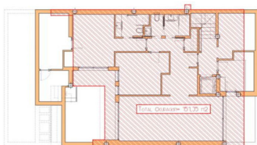
PLANTA SOTANO
