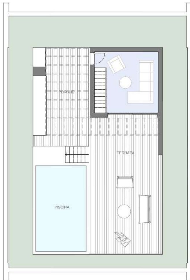
PLANTA CUBIERTA
