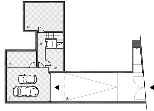
PLANTA SÓTANO / BASEMENT FLOOR
