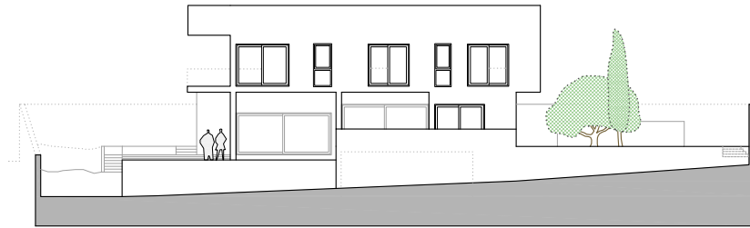
ALZADO ESTE / EAST ELEVATION
