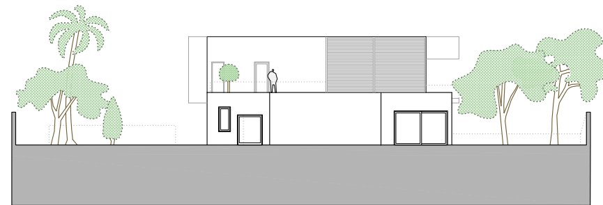
ALZADO OESTE / WEST ELEVATION
