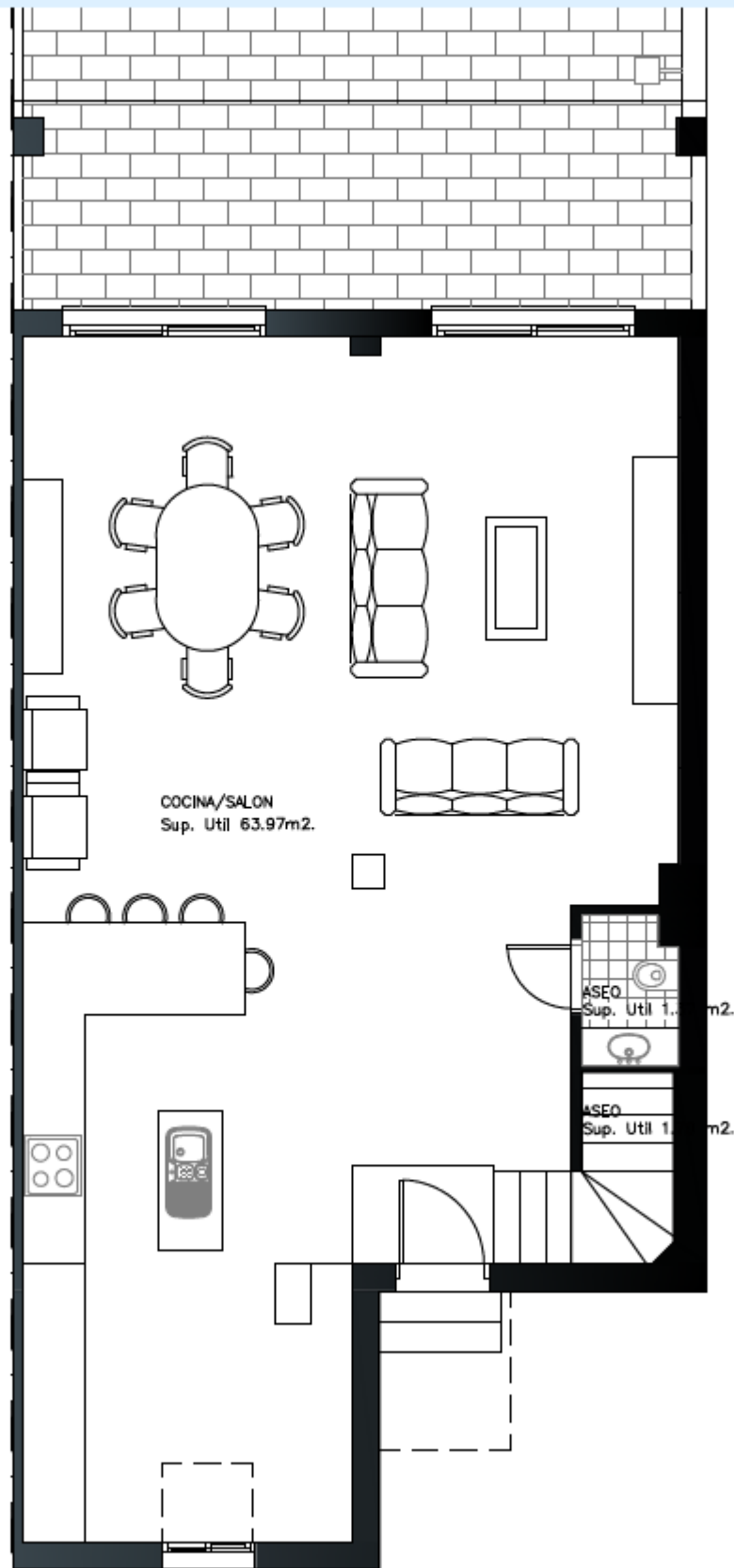
PLANTA BAJA DISTRIBUCION
