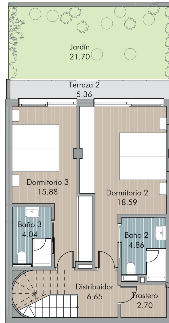
PLANTA SEGUNDA
