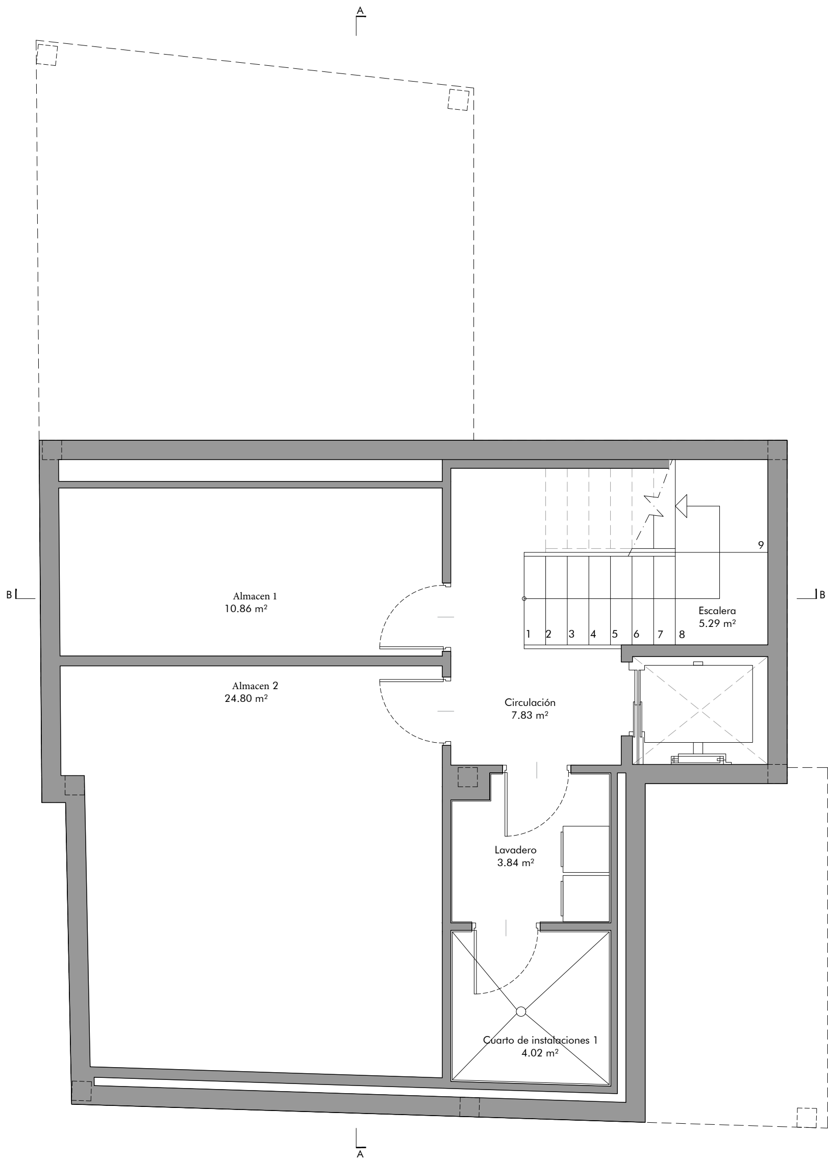
PLANTA SÓTANO
