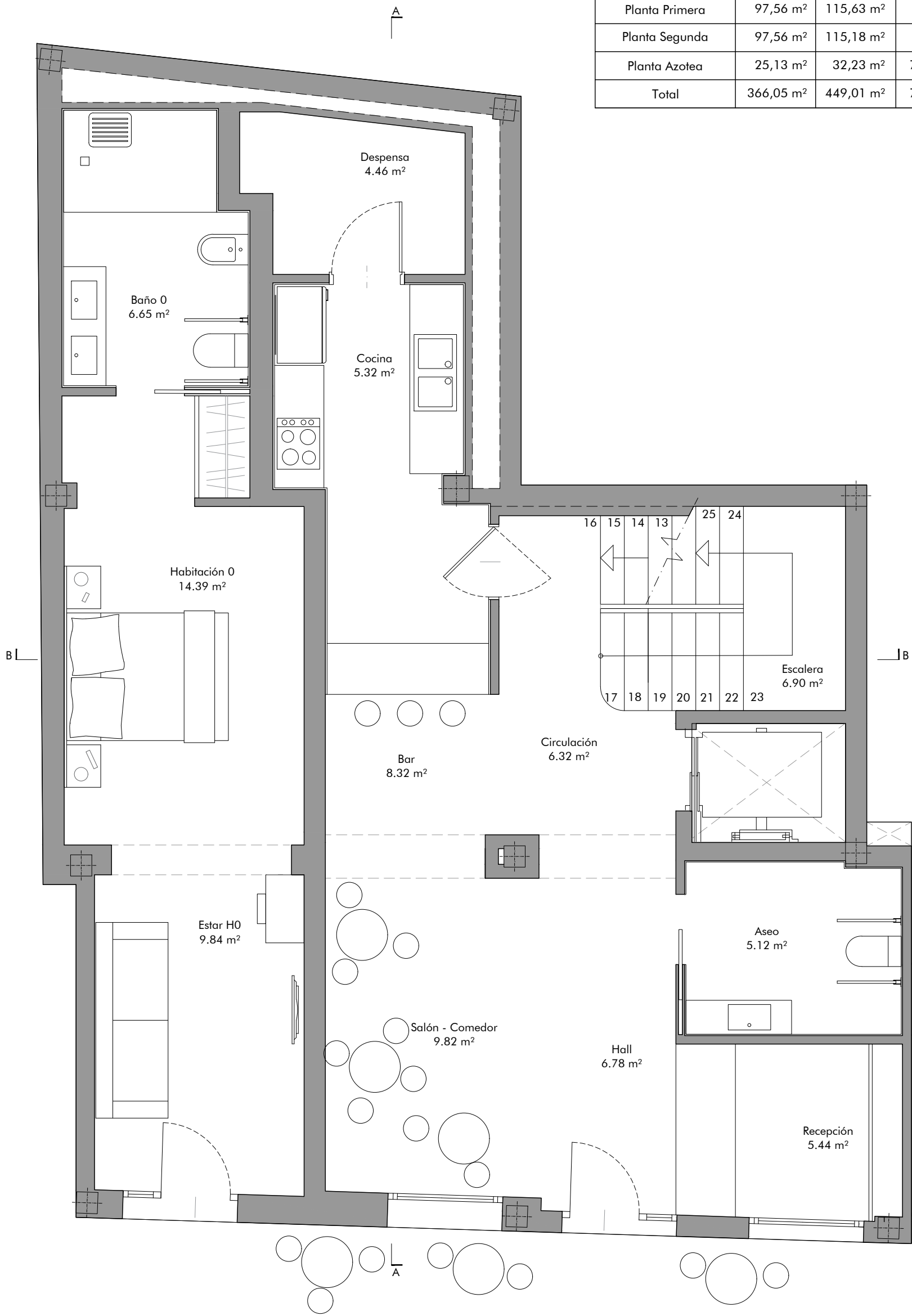
PLANTA BAJA
