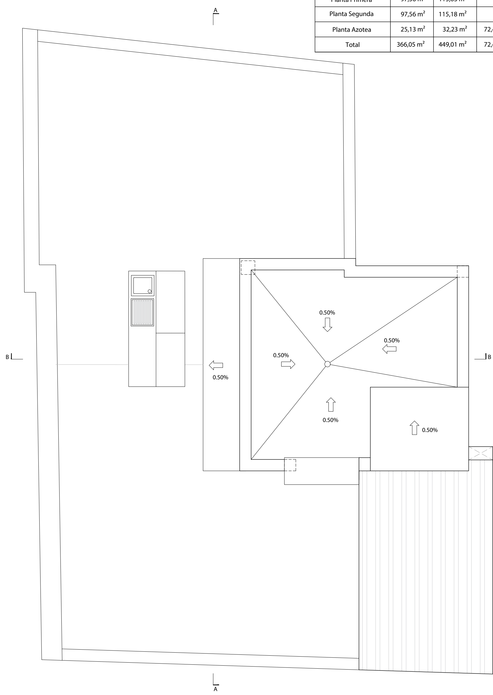
CUBIERTA
