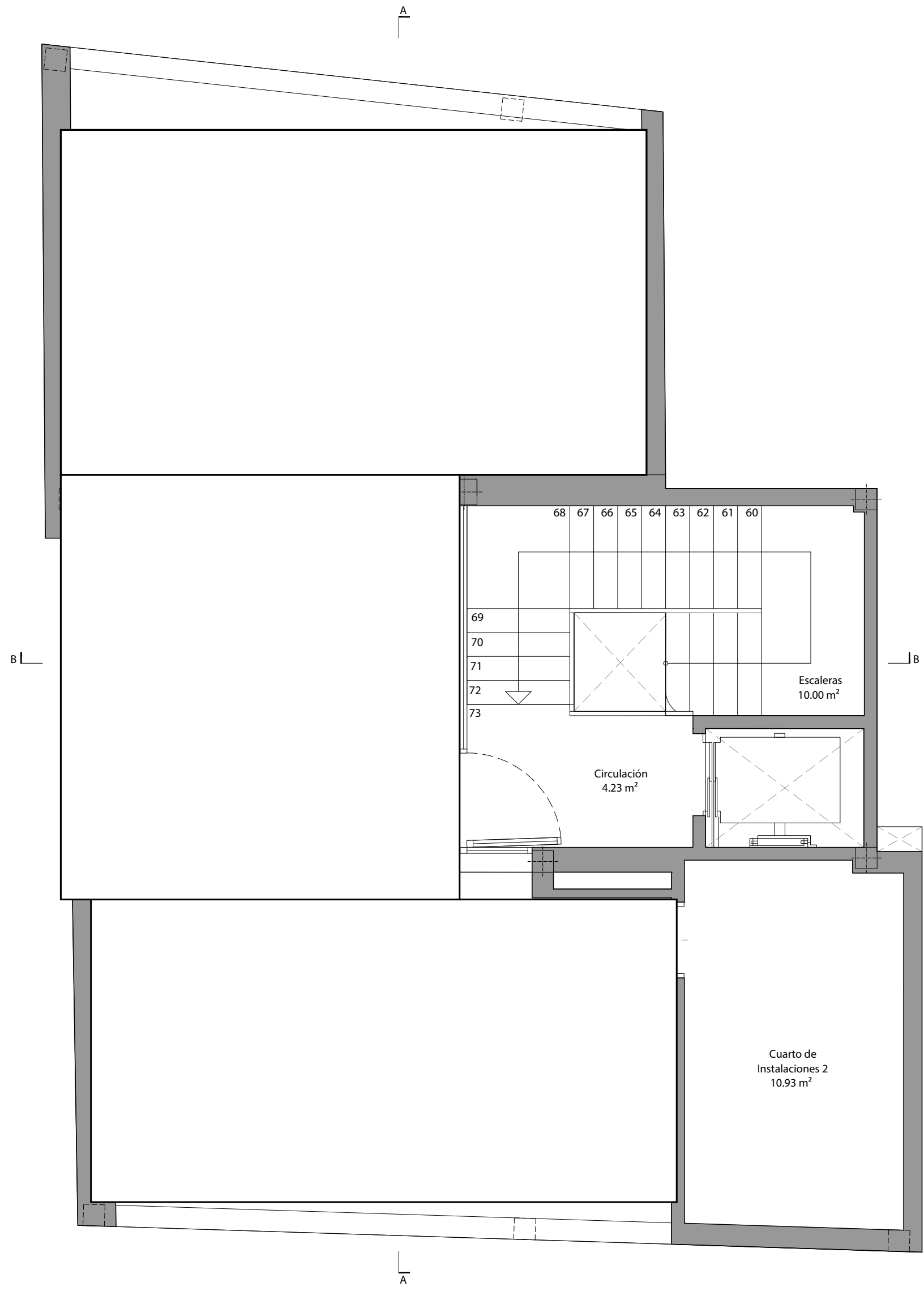
PLANTA TERCERA
