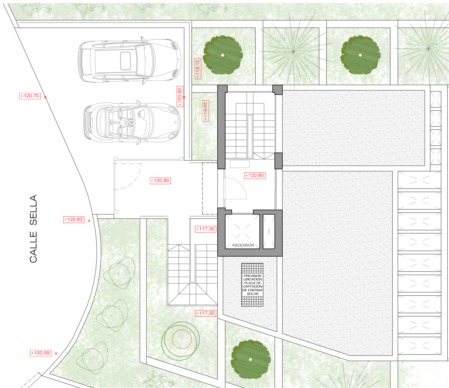
PLANTA ACCESO CALLE
