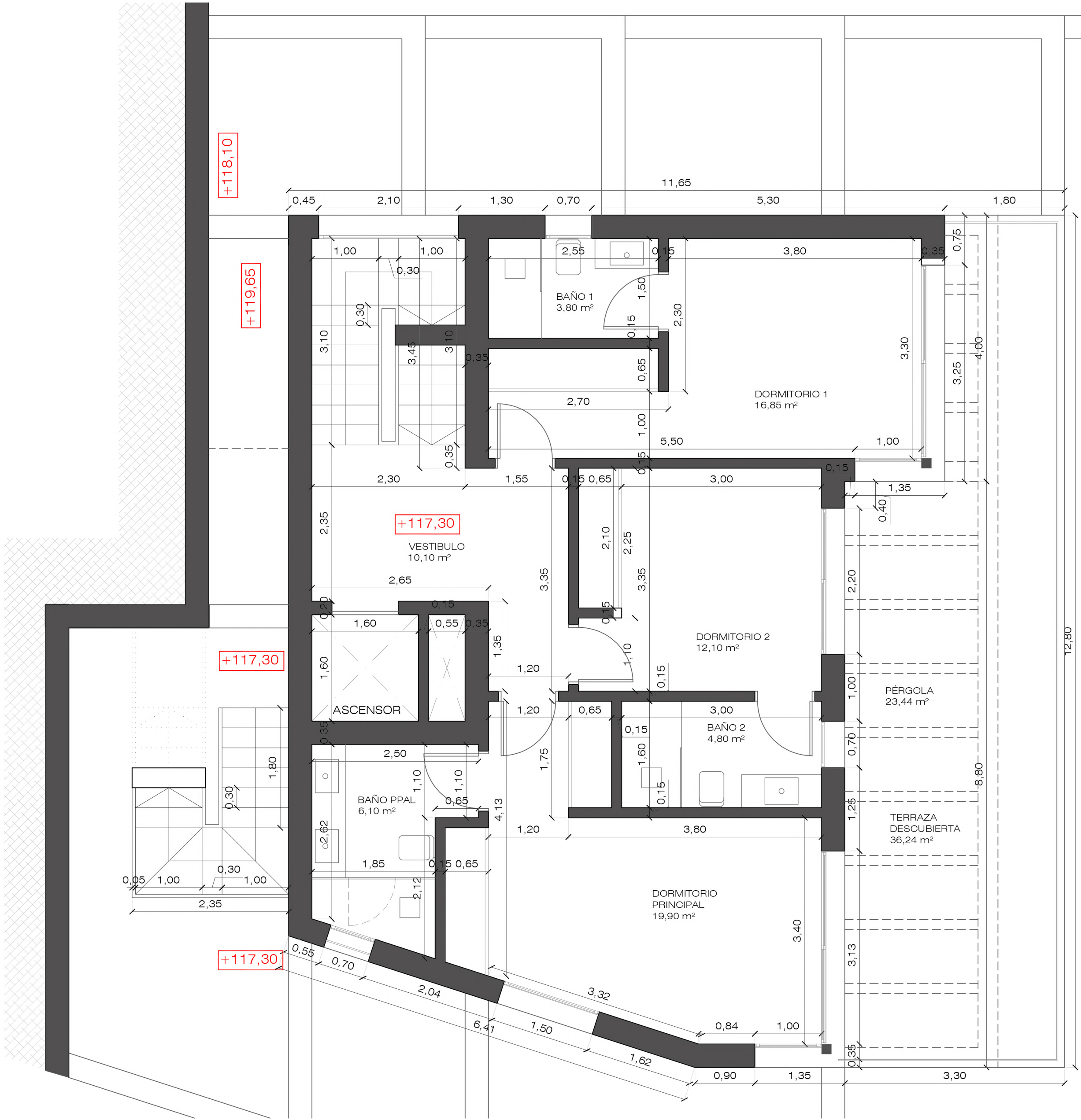
PLANTA ALTA
