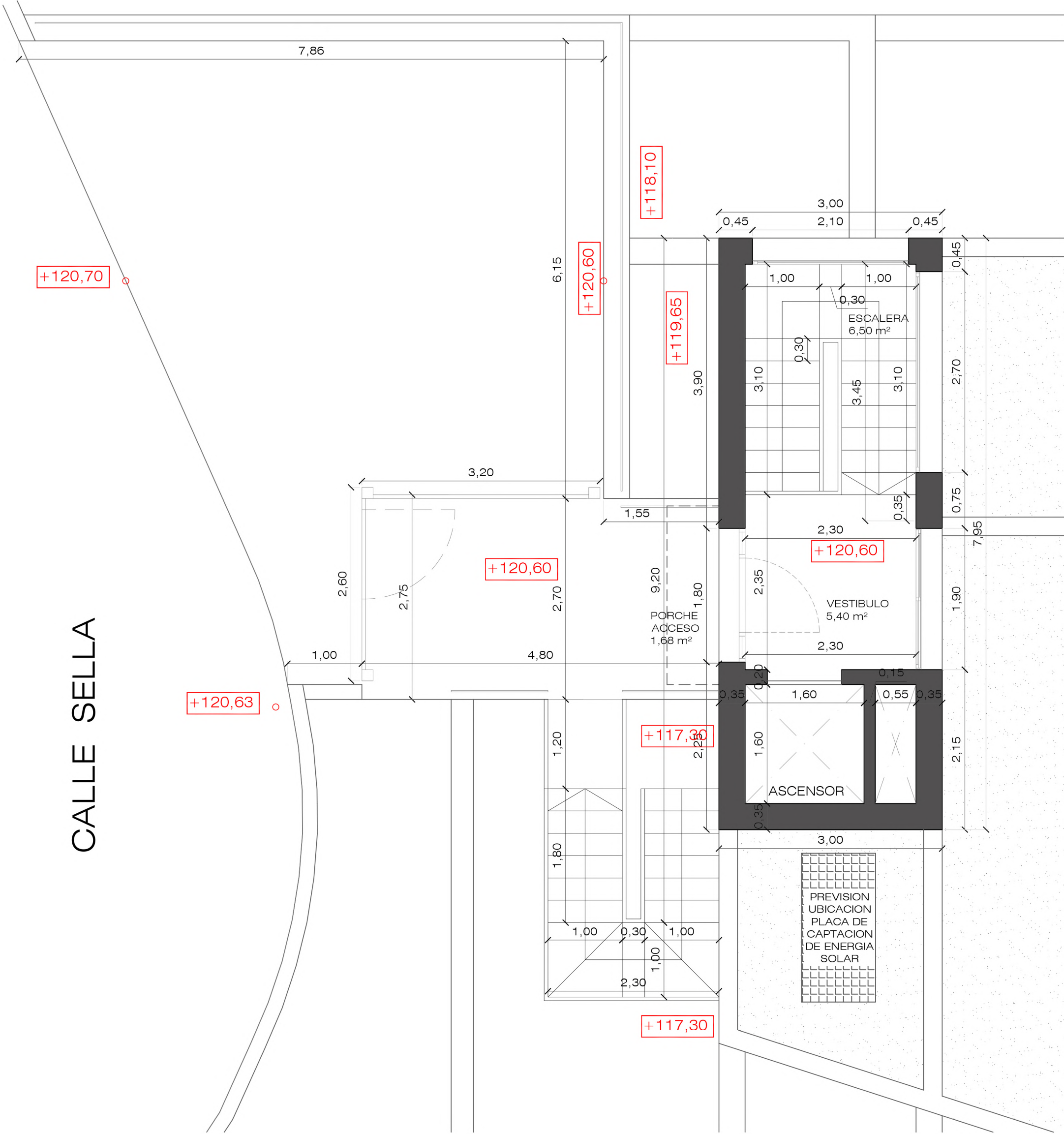
PLANTA ACCESO
