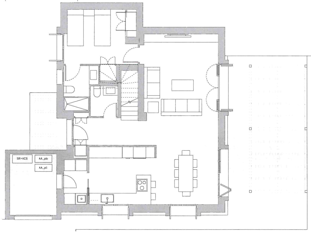
Planta baja
