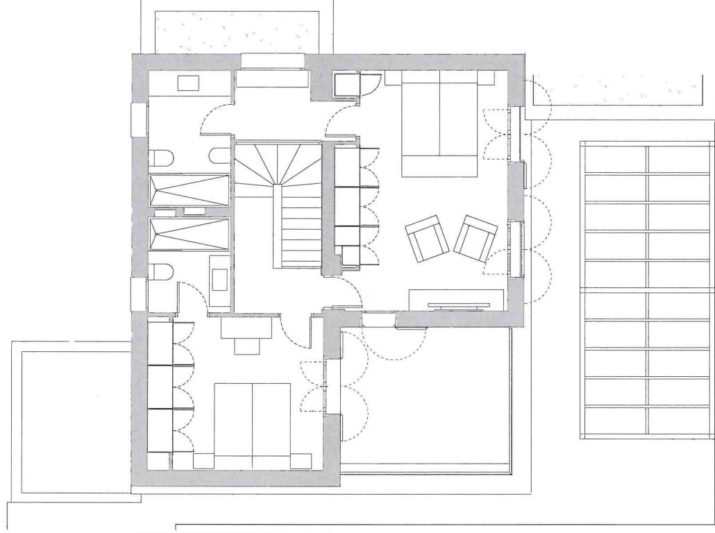
Planta primera
