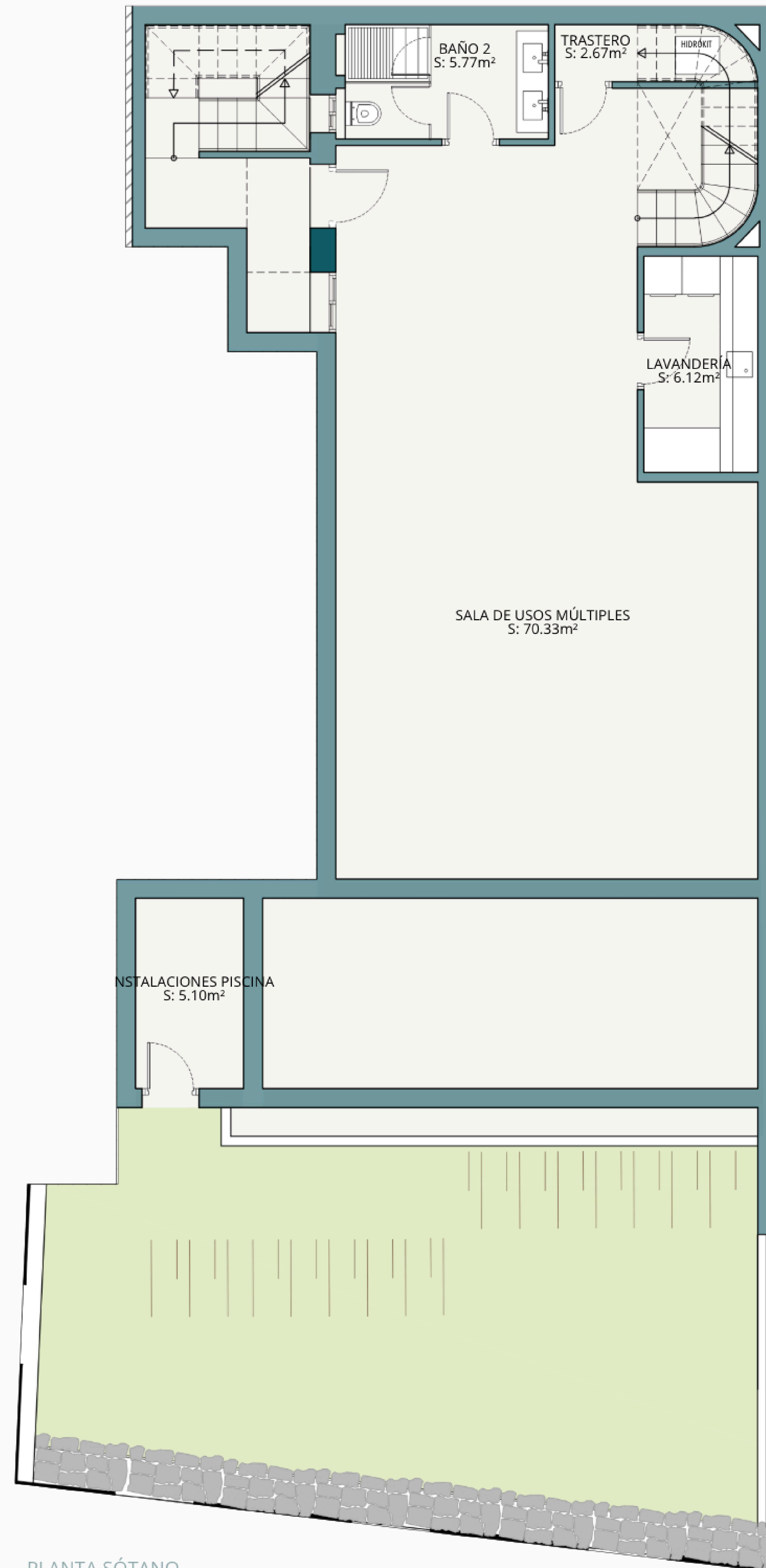
PLANTA SÓTANO
