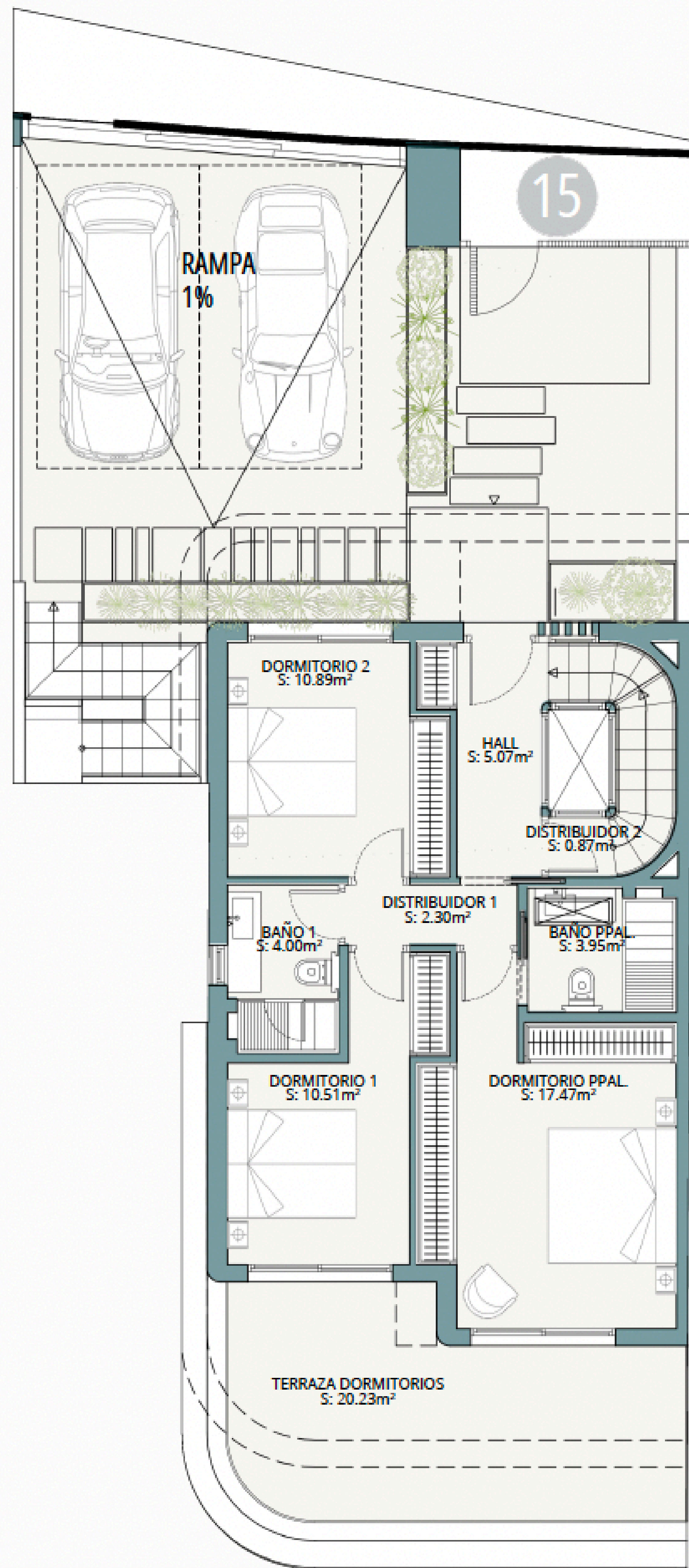
PLANTA PRIMERA
