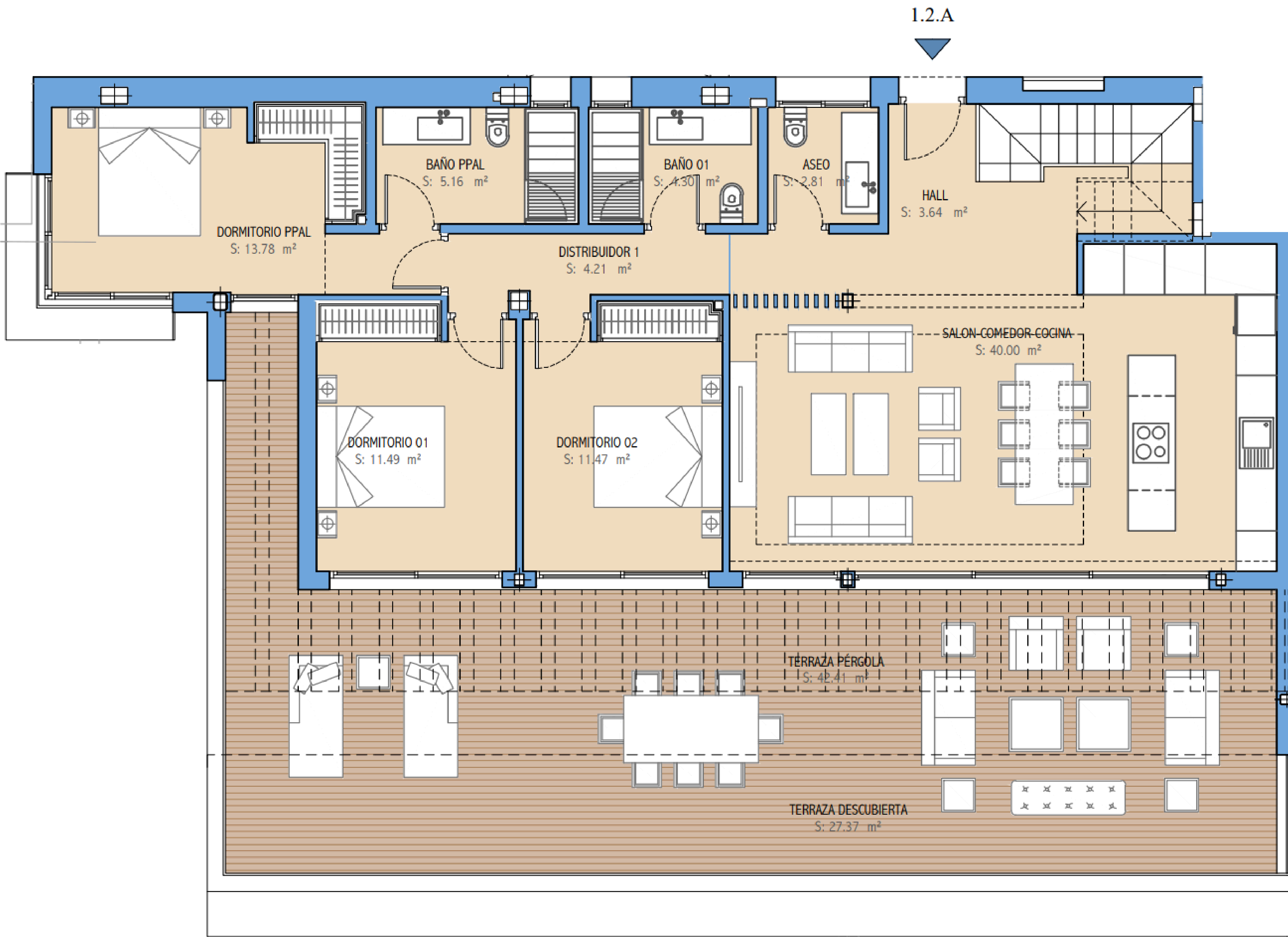
PLANTA ÁTICO
