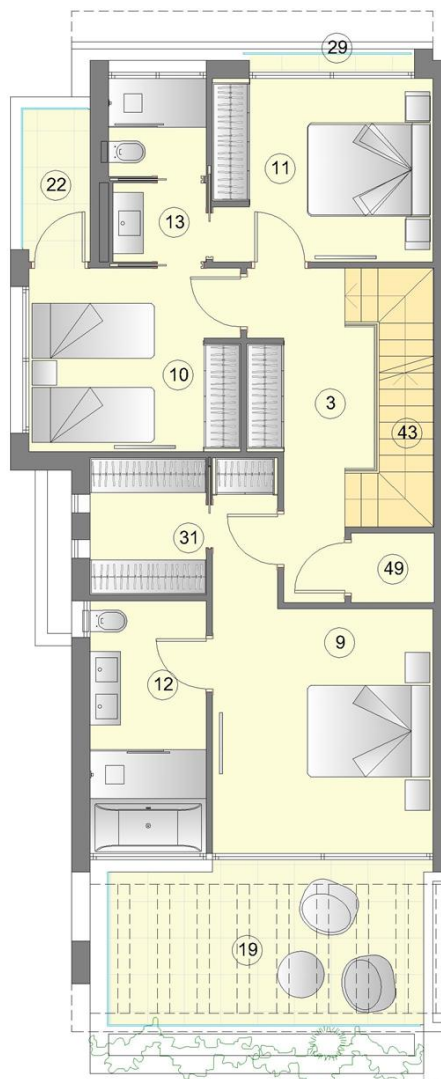
PLANTA PRIMERA
