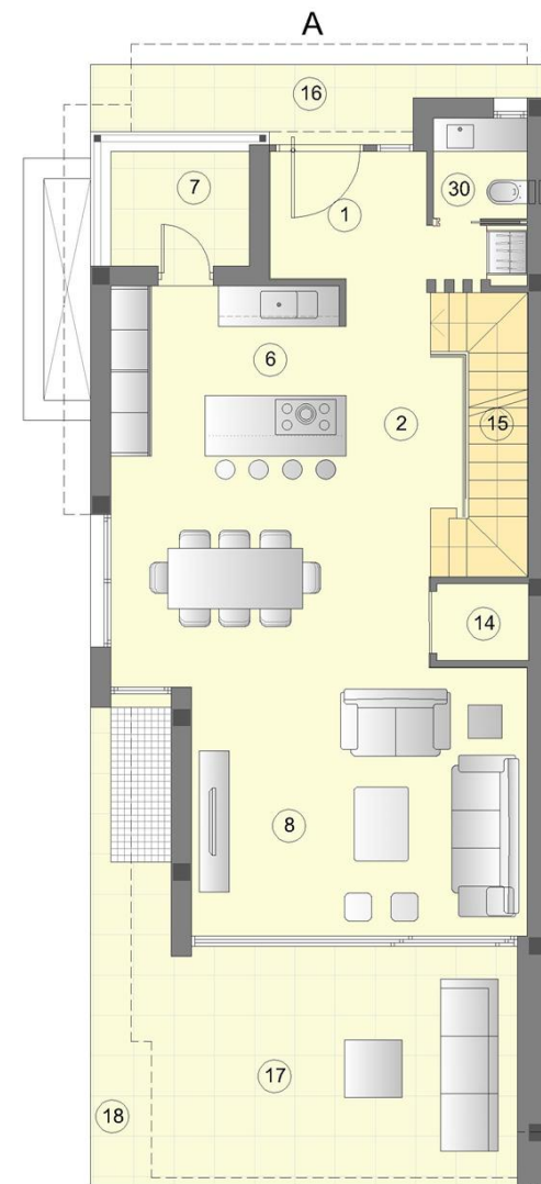
PLANTA BAJA
