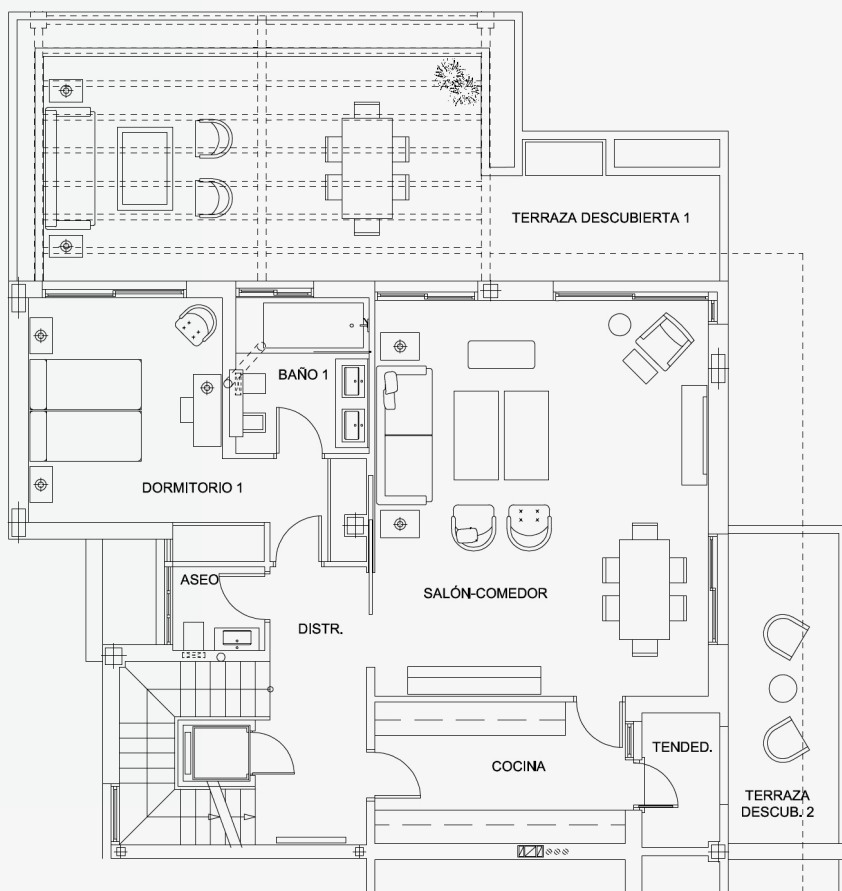
PLANTA ALTA
