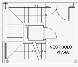
PLANTA BAJA
