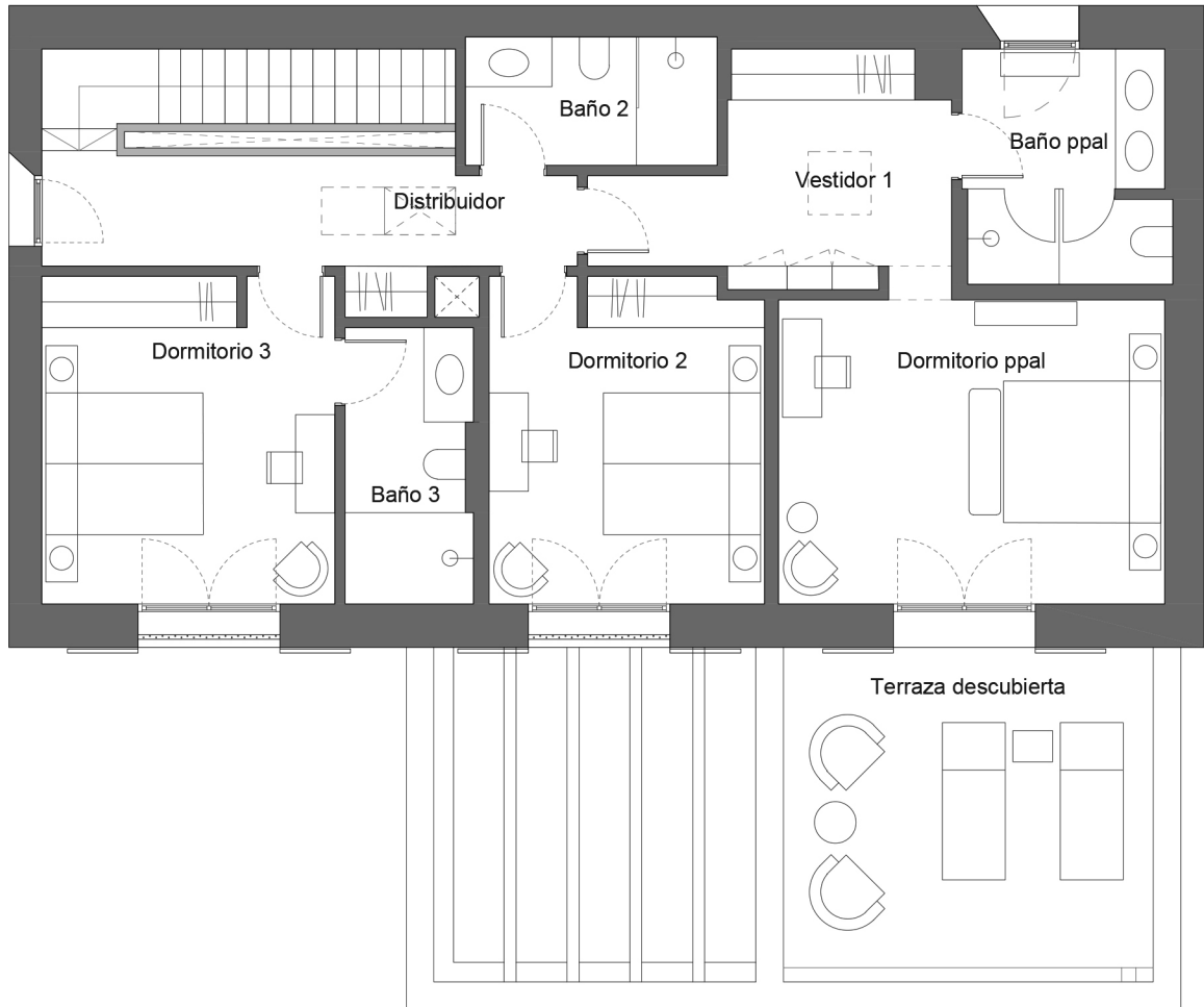
Planta Primera
